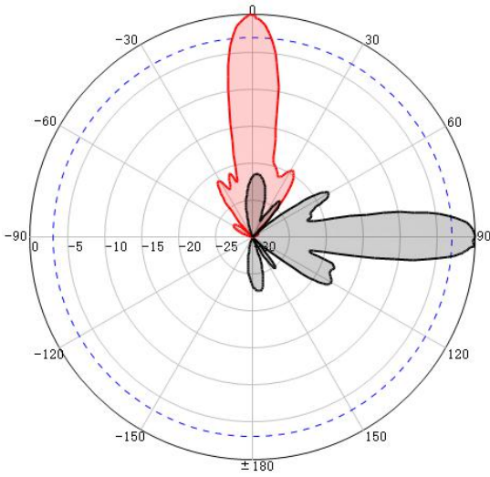
H-Pol@2700MHz
