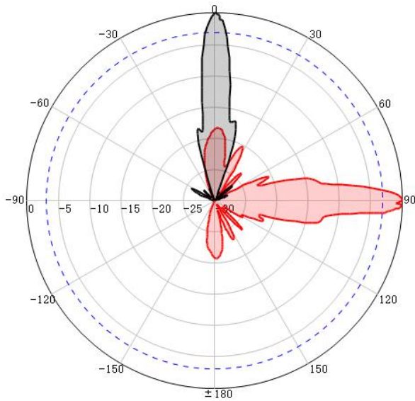
H-Pol@3500MHz
