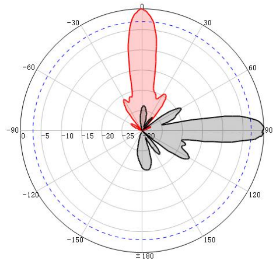
V-Pol@2700MHz
