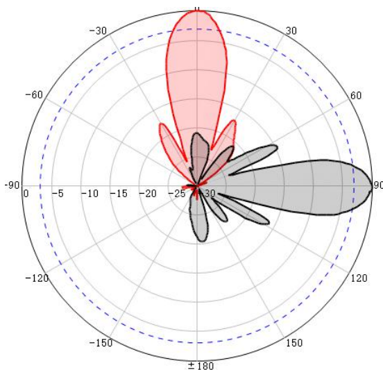
H-Pol@1710MHz
