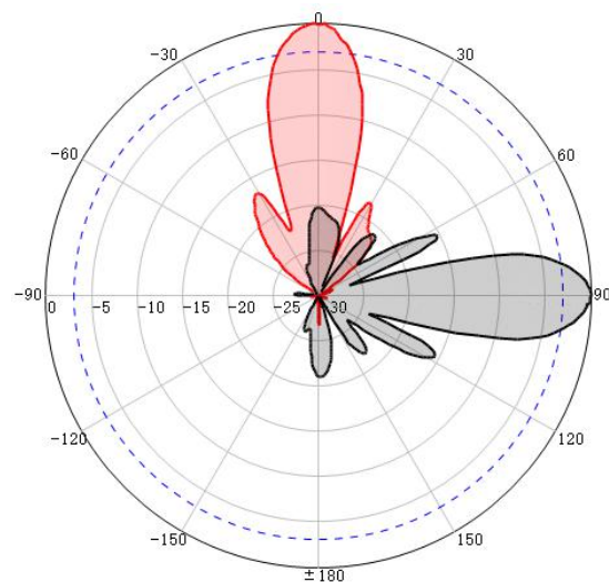
V-Pol@1710MHz
