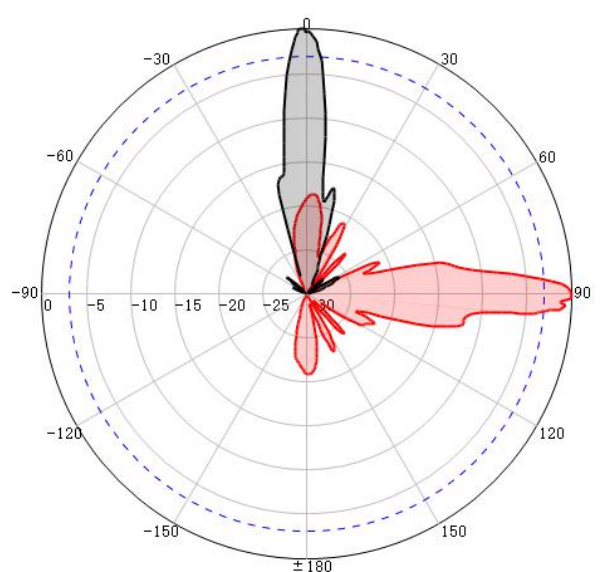
V-Pol@3500MHz
