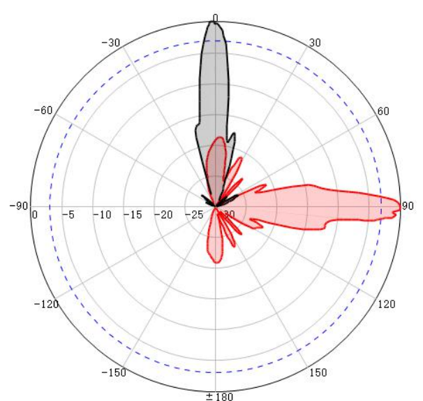
V-Pol@3500MHz
